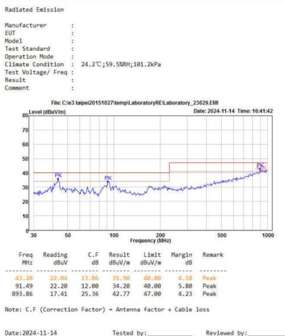
图 5-7 辐射测试垂直方向
