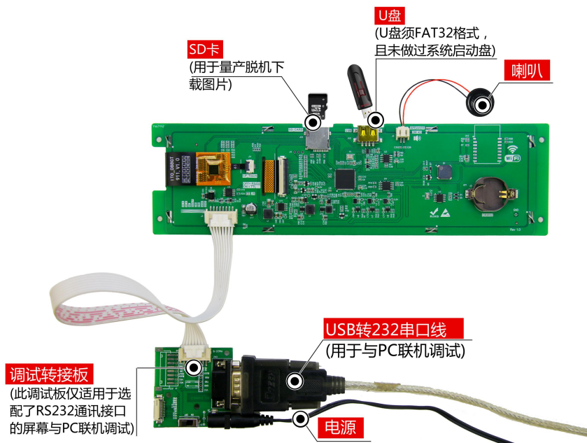
图 1-3 调试工具图
