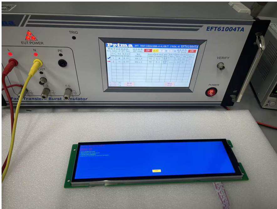
图 5-4 群脉冲测试图
